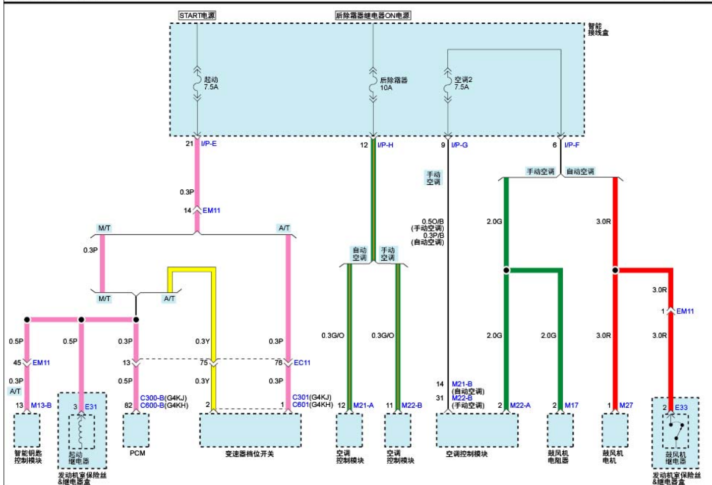
室内保险丝分布(8)
